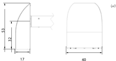
CONTURA DLA BASENU O SZEROKOŚCI DO 5 m
