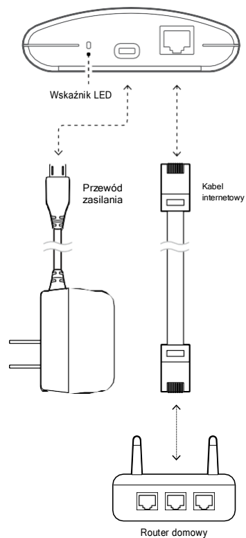
Moduł GATEWAY ULTRA (widok z boku)
