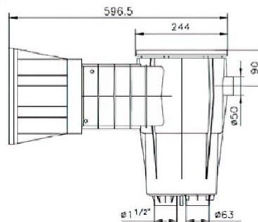
Wymiary skimmera z dużym otworem
