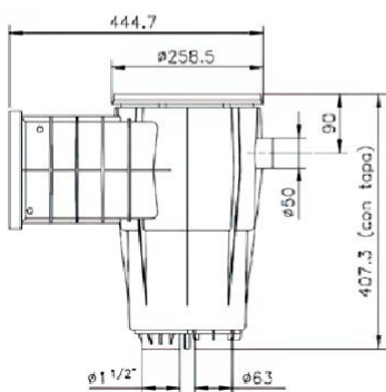
Wymiary skimmera z małym otworem
